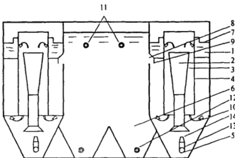
Рис. 8. Осветлитель-рециркулятор:
