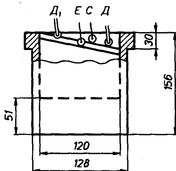
Рисунок 1 — Зональный пробоотборник
