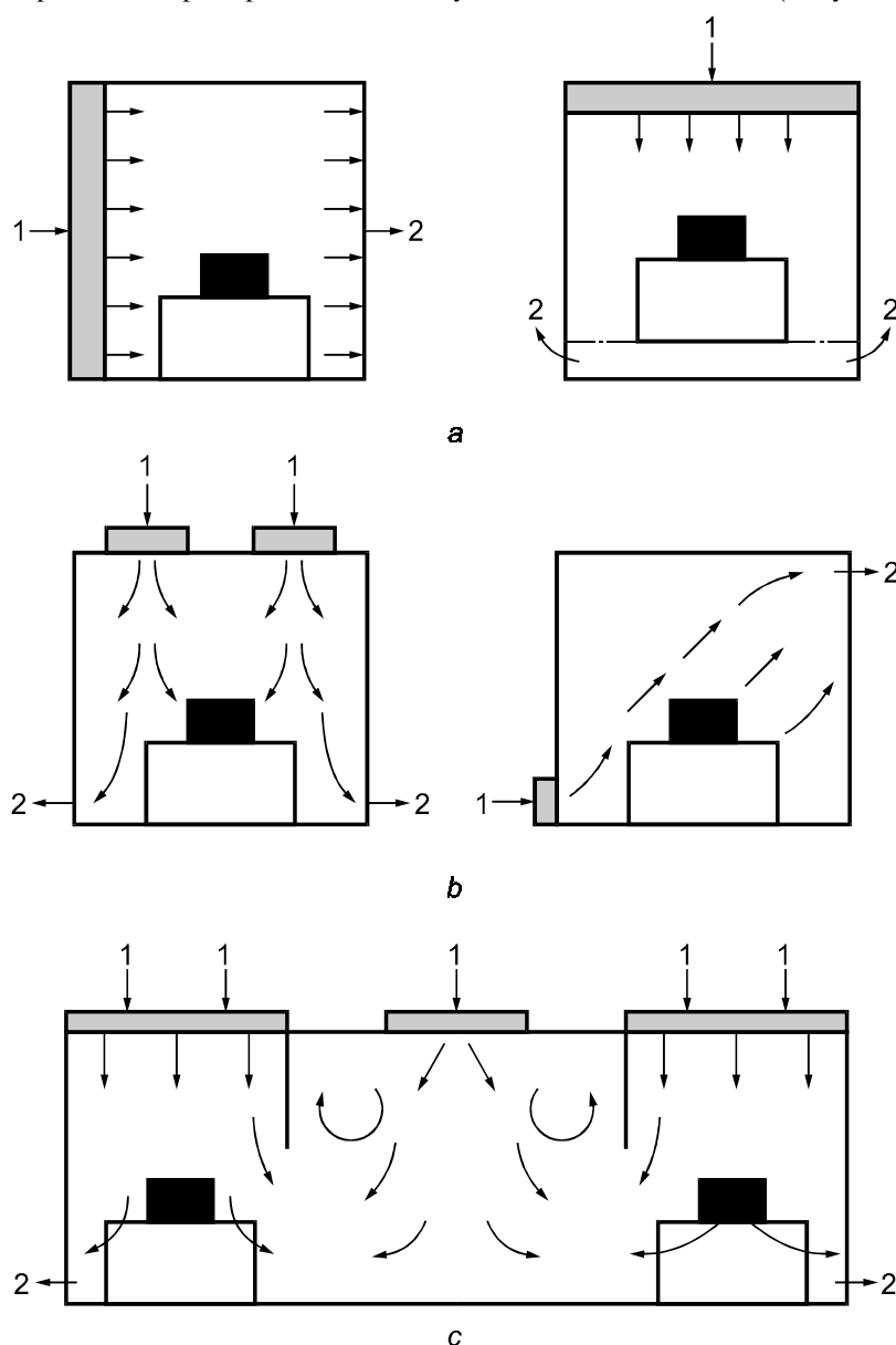
a — однонаправленный поток воздуха; b — неоднаправленный поток воздуха; c — смешанный поток воздуха; 1 — приточный воздух; 2 — вытяжной воздух
